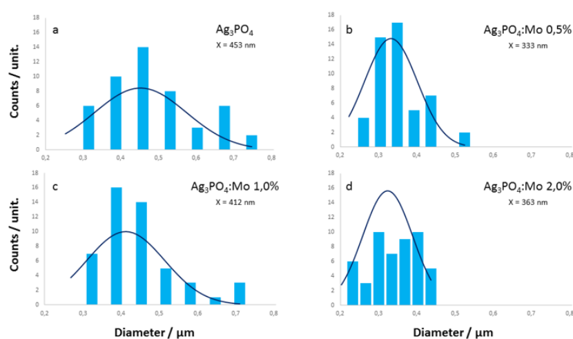
Figure SI-6. Size distribution for \text{Ag}_3\text{PO}_4 (a), \text{Ag}_3\text{PO}_4:\text{Mo} 0.5% (b), \text{Ag}_3\text{PO}_4:\text{Mo} 1% (c) and \text{Ag}_3\text{PO}_4:\text{Mo} 2% (d) particles.
