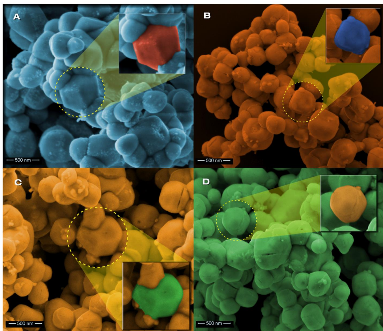
Figure 5 - FEG-SEM images of (a) \text{Ag}_3\text{PO}_4 , (b) \text{Ag}_3\text{PO}_4:\text{Mo} 0.5%, (c) \text{Ag}_3\text{PO}_4:\text{Mo} 1% and (d) \text{Ag}_3\text{PO}_4:\text{Mo} 2%.
