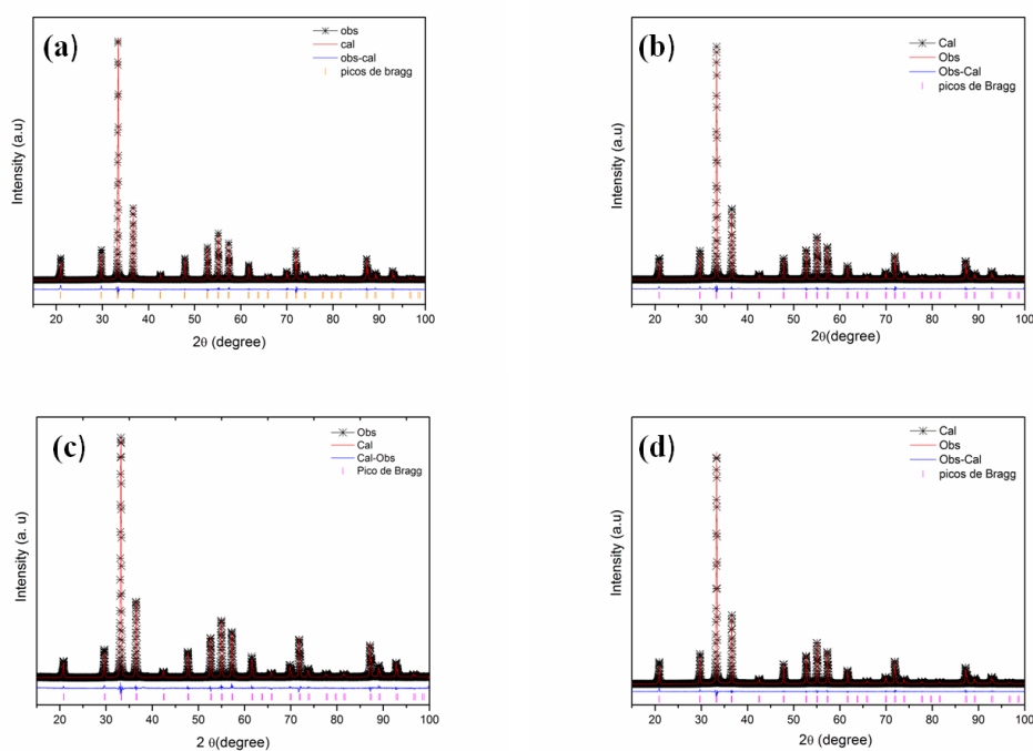
Figure SI-2. Rietveld refinement plots of pure \text{Ag}_3\text{PO}_4 (a), \text{Ag}_3\text{PO}_4:\text{Mo} 0.5% (b), \text{Ag}_3\text{PO}_4:\text{Mo} 1% (c) and \text{Ag}_3\text{PO}_4:\text{Mo} 2% (d).
