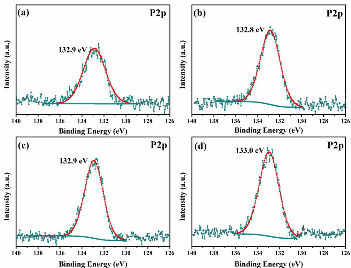
Figure SI-5. XPS spectrum of P 2p for pure \text{Ag}_3\text{PO}_4 (a), \text{Ag}_3\text{PO}_4:\text{Mo} 0.5% (b), \text{Ag}_3\text{PO}_4:\text{Mo} 1% (c) and \text{Ag}_3\text{PO}_4:\text{Mo} 2% (d) samples.
