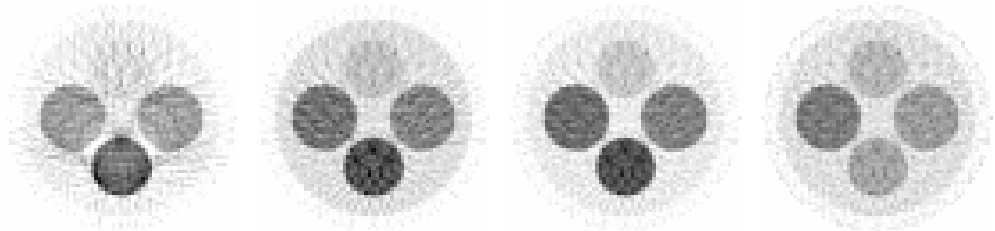
FIGURA 5.4 - Imagens adquiridas com energias de 40, 60, 85 e 662 keV.
