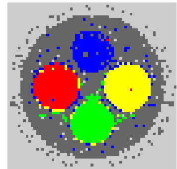
Decision Templates Erro: 0,0375 / Kappa: 0,9550
