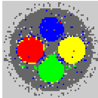
Bagging c/ Decision Templates Erro: 0,0208 / Kappa: 0,9750
