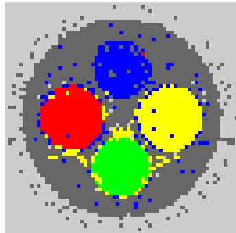
Dempster-Shafer Erro: 0,0292 / Kappa: 0,9650
