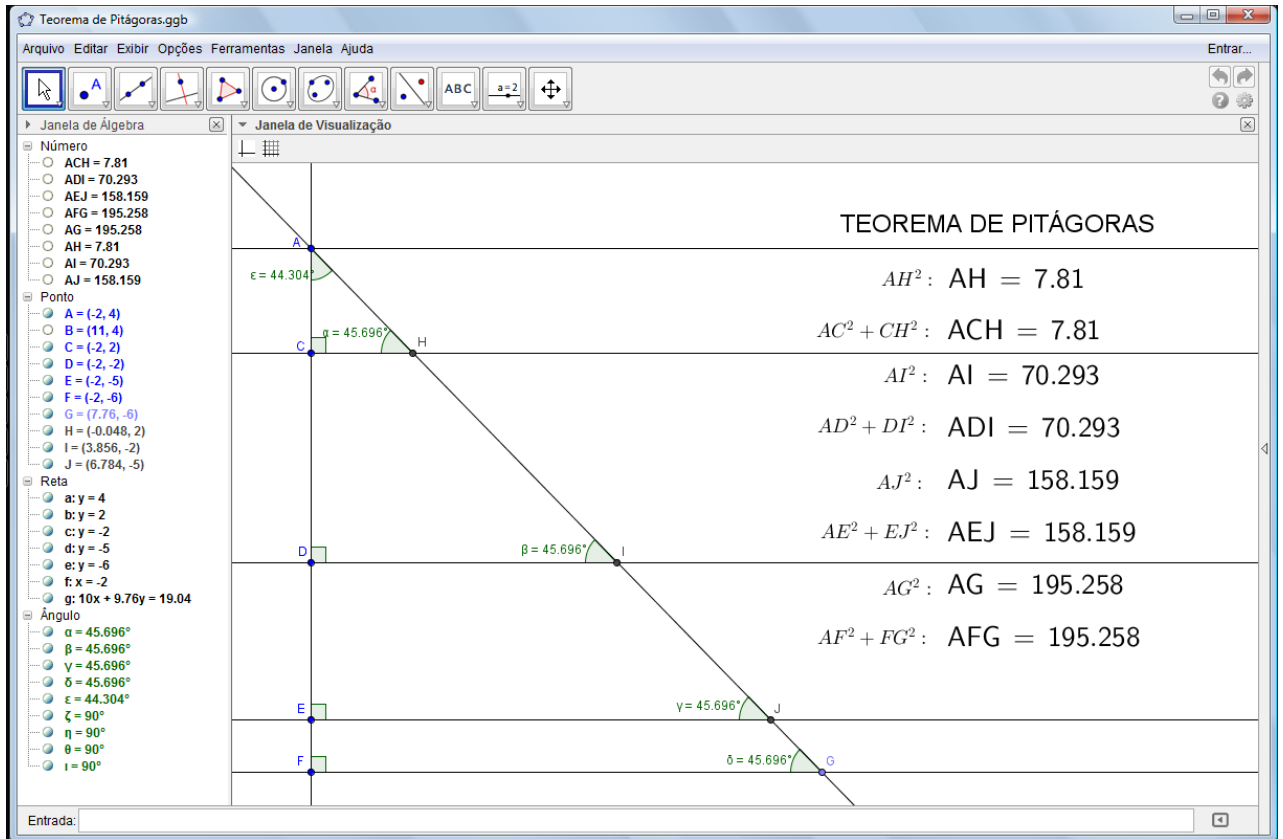
Figura 6: Atividade no GeoGebra sobre Teorema de Pitágoras.
