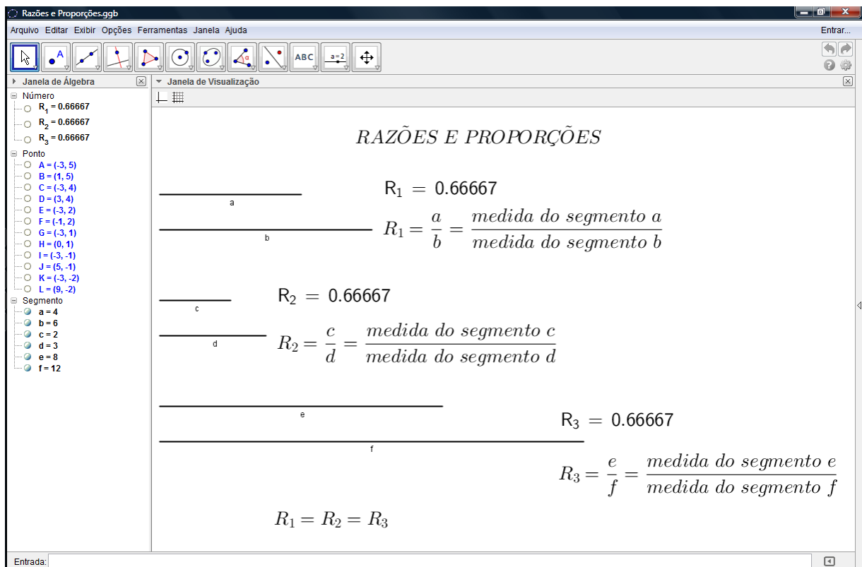
Figura 1: Atividade no GeoGebra sobre Razões e Proporções.
