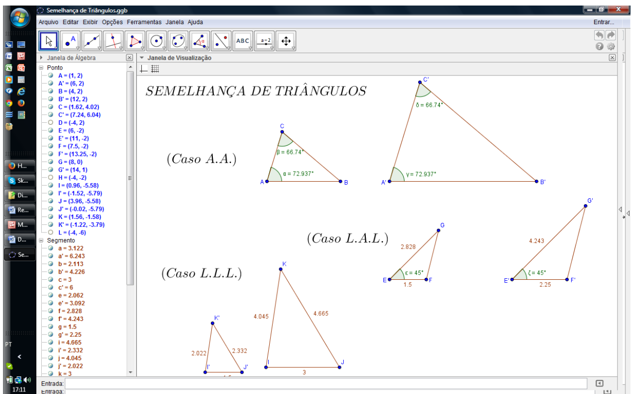
Figura 5: Atividade no GeoGebra sobre semelhança de triângulos.
