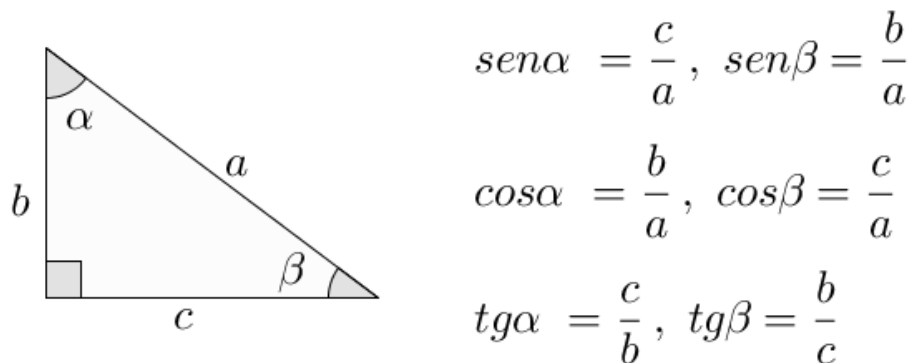
Figura 7: Razões trigonométricas como apresentadas em sala de aula.
