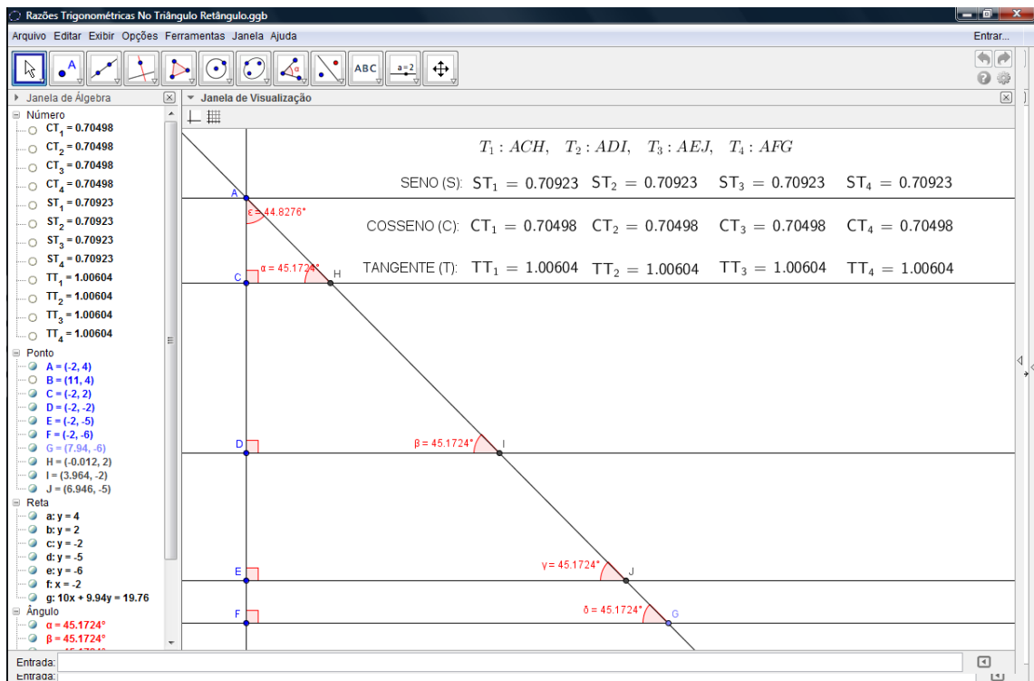
Figura 8: Atividade no GeoGebra sobre razões trigonométricas.
