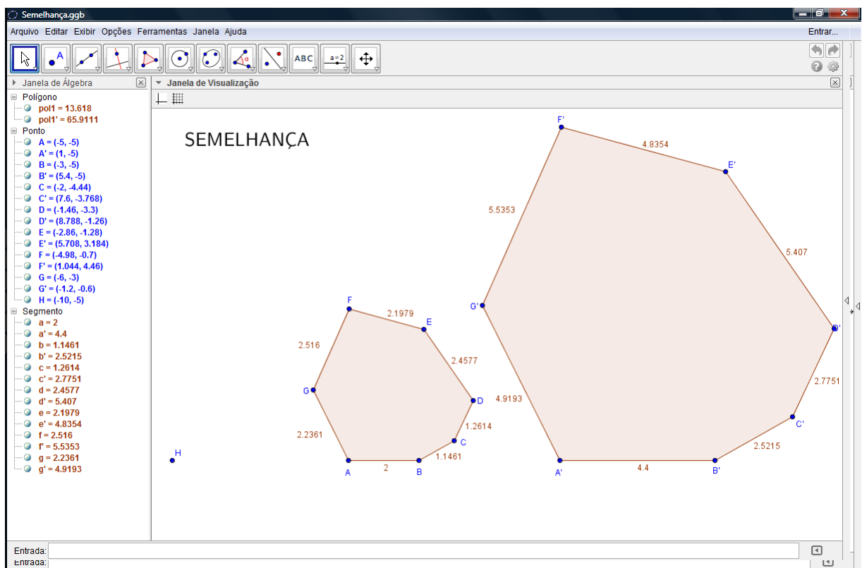
Figura 4: Atividade no GeoGebra sobre semelhança.
