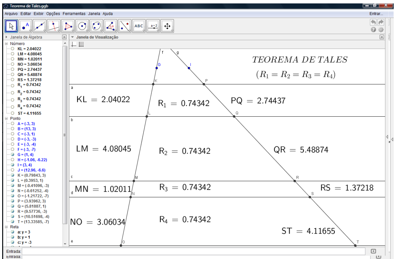
Figura 3: Atividade no GeoGebra sobre Teorema de Tales.
