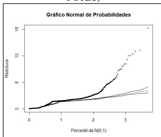
Figura 2 - Envelope plot dos resíduos de Pearson do modelo de Poisson (mobilidade POTEÇ)
