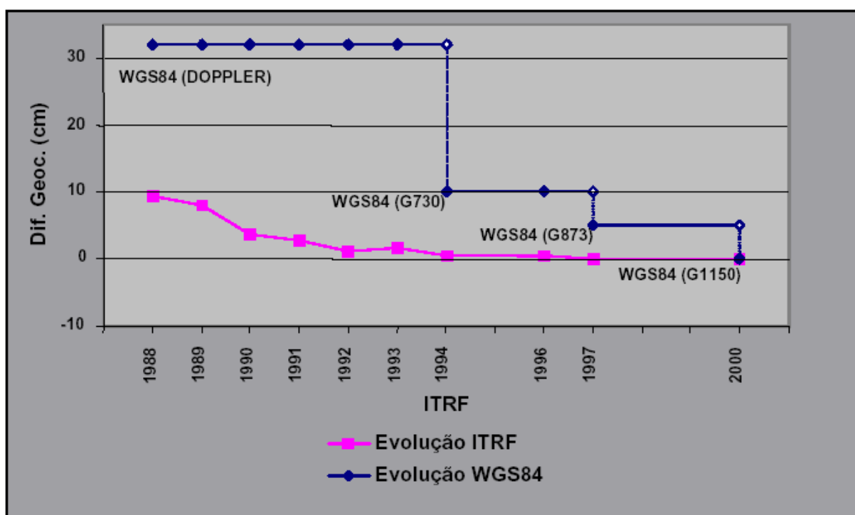
Figura 2.18 – Evolução do WGS-84 aproximando do ITRF ao longo do tempo
