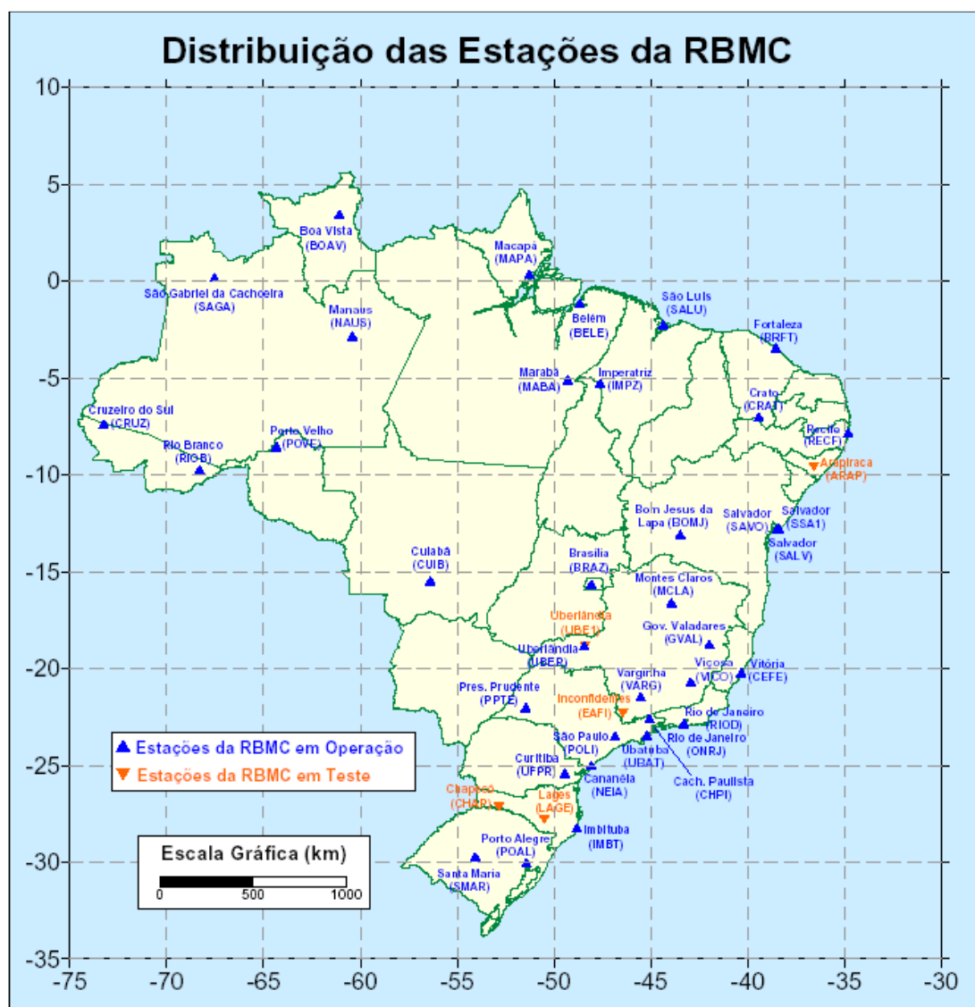
Figura 2.2 – Cartograma das Estações da RBMC
