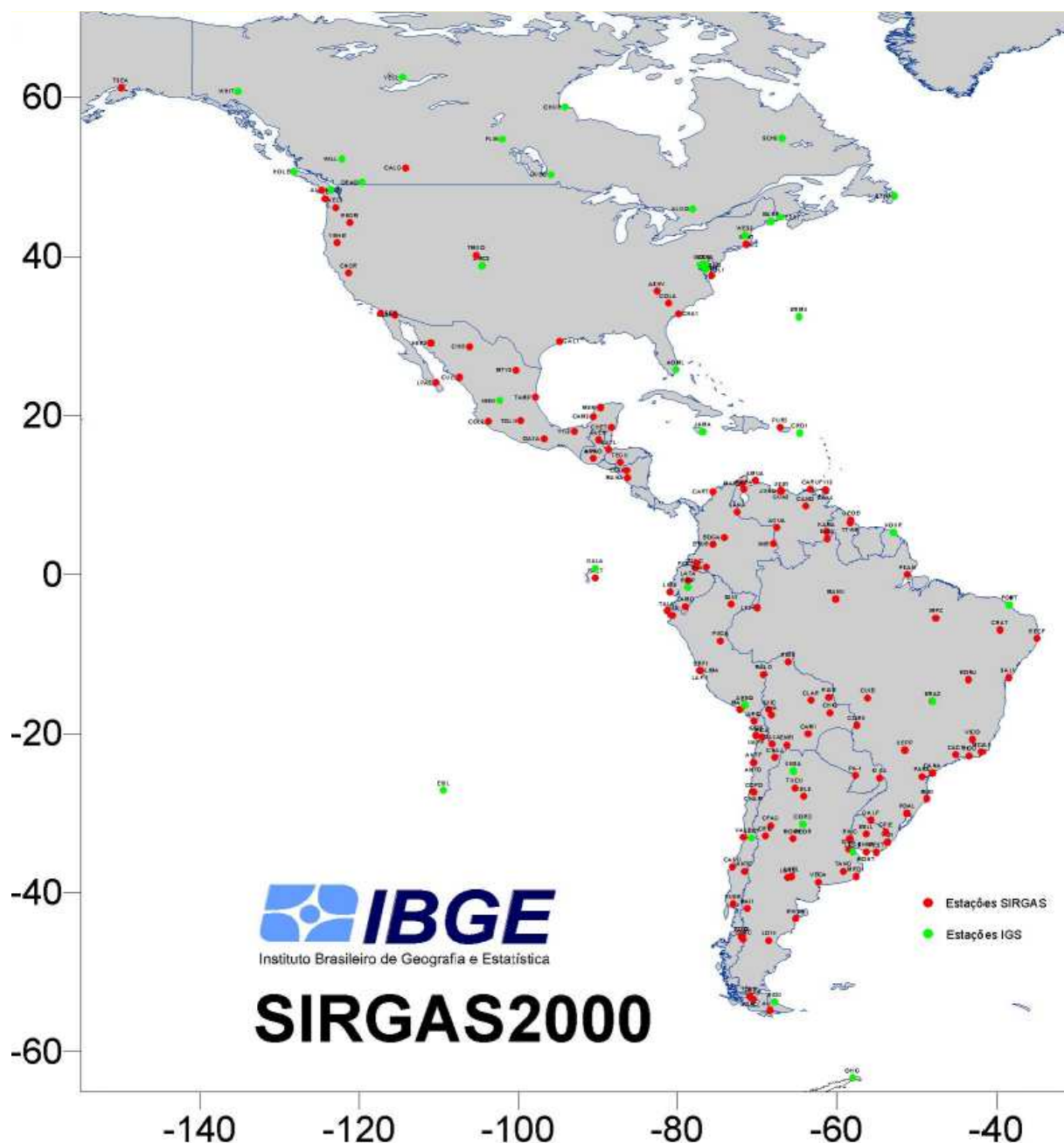
Figura 2.10 - Rede de Estações SIRGAS e IGS
