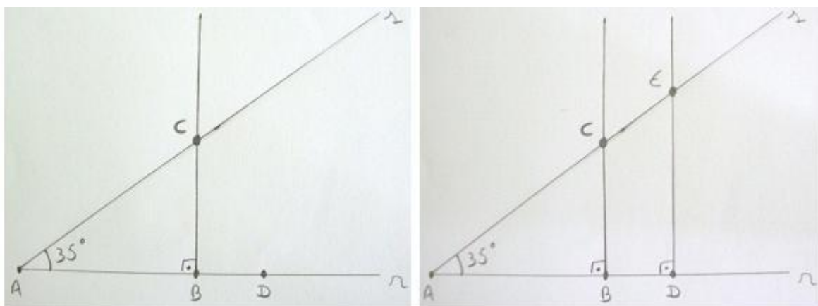
Figura 6 Construção do triângulo retângulo ADE
