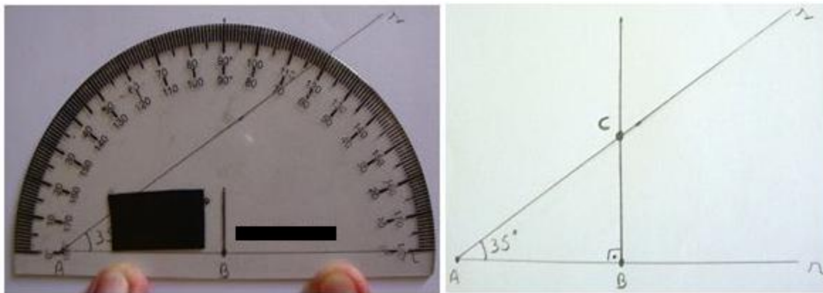
Figura 5 Construção do ângulo reto e da semirreta perpendicular
