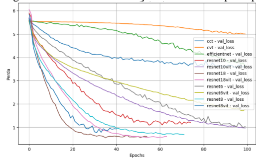
Figura 11 - Perda na Validação Multiclasses por Época.
