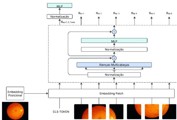
Figura 5 – Arquitetura do Vision Transformer.
