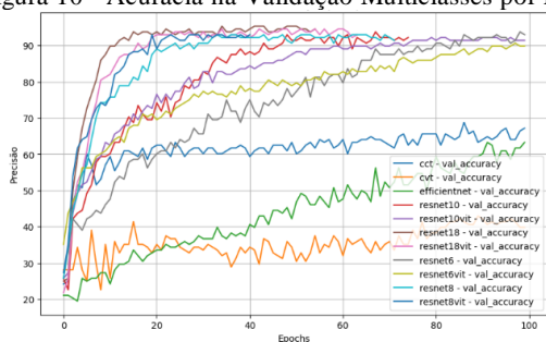
Figura 10 - Acurácia na Validação Multiclasses por Época.
