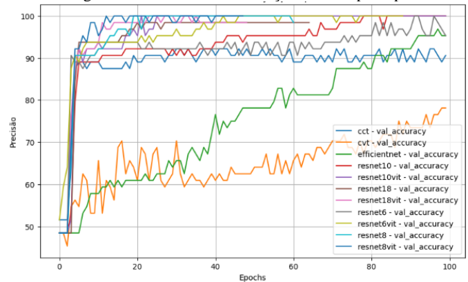
Figura 7 - Acurácia na Validação Binária por Época.
