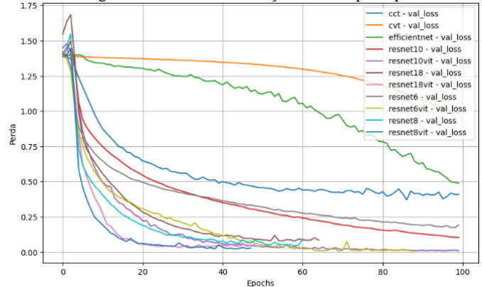
Figura 8 - Perda na Validação Binária por Época.
