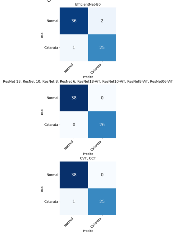
Figura 9 -Matriz confusão binária.
