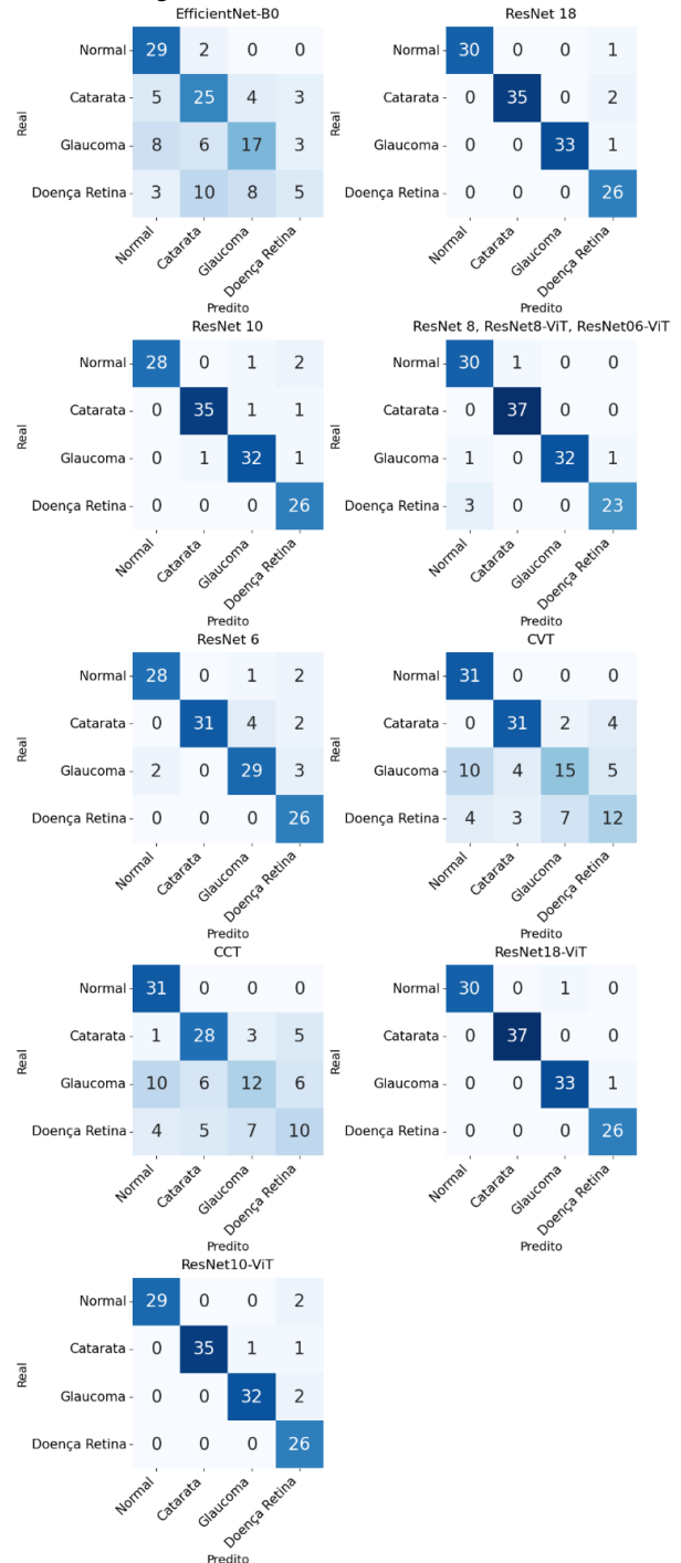
Figura 12 – Matriz confusão multiclasses.
