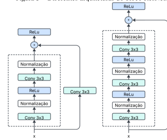
Figura 3 – Diferentes arquiteturas do bloco ResNet.
