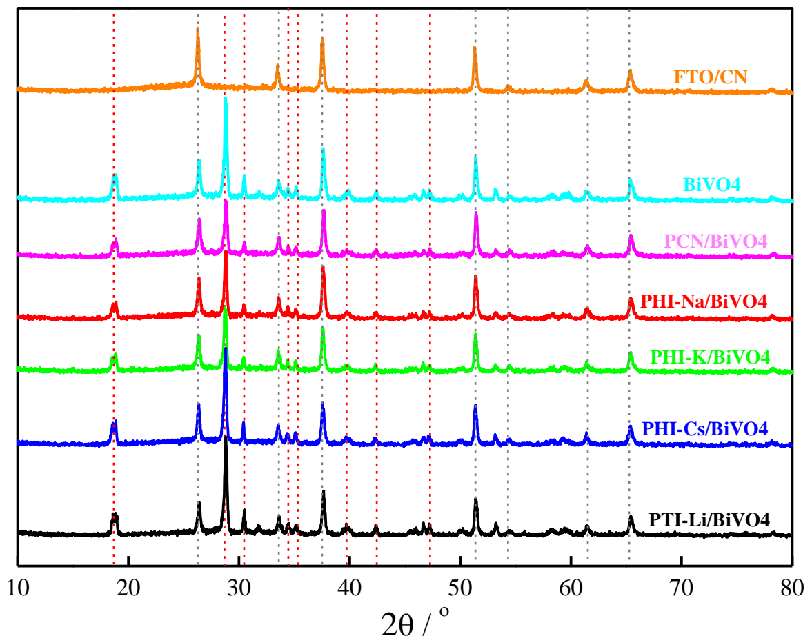
FIGURA 4.6 - Difratograma de Raios-X para os materiais de FTO, \text{BiVO}_4 , \text{PCN}/\text{BiVO}_4 , \text{Na-PHI}/\text{BiVO}_4 , \text{K-PHI}/\text{BiVO}_4 , \text{Cs-PHI}/\text{BiVO}_4 e \text{Li-PTI}/\text{BiVO}_4 .
