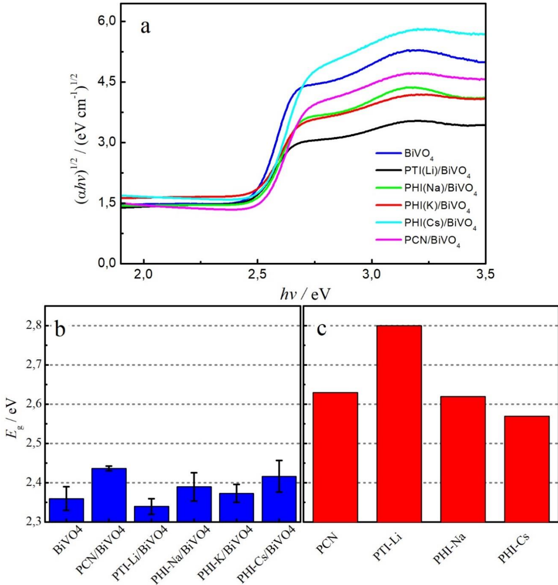
FIGURA 4.8 - (a) Gráfico de Tauc para os filmes sintetizados: \text{BiVO}_4 , \text{PCN/BiVO}_4 , \text{Na-PHI/BiVO}_4 , \text{K-PHI/BiVO}_4 , \text{Cs-PHI/BiVO}_4 e \text{Li-PTI/BiVO}_4 ; (b) energia de bandgap ( E_g ) para os filmes mostrados em (a); (c) E_g para os nitretos de carbono na forma de pós.
