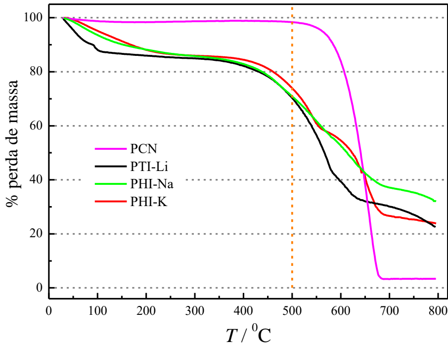
FIGURA 4.1 - Análise termogravimétrica dos materiais de nitretos de carbono: nitreto de carbono polimérico (PCN), poli (triazina imida) de lítio (Li-PTI), poli (heptazina imida) de sódio (Na-PHI) e poli (heptazina imida) de potássio (K-PHI).
