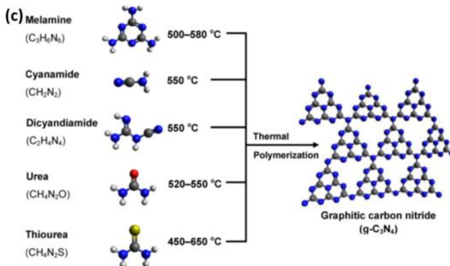
FIGURA 1.3 - Polimerização térmica de diferentes precursores para sínteses de nitreto de carbono.
