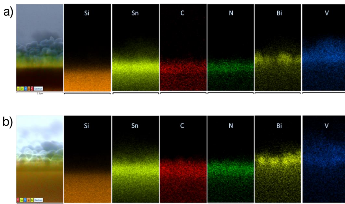
FIGURA 4.5 - Mapeamento cross-section EDS para os eletrodos de a) PCN/ \text{BiVO}_4 ; b) Li-PTI/ \text{BiVO}_4 .
