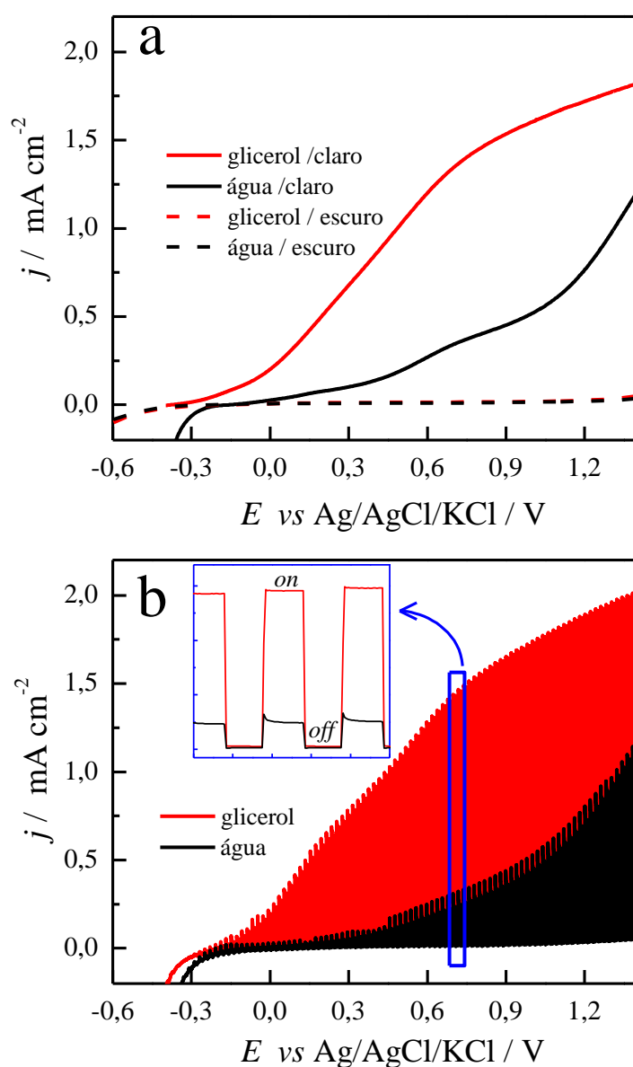
FIGURA 4.10 - Voltamogramas lineares na ausência e presença de iluminação contínua (a) e iluminação intermitente (b) para os filmes de BiVO_4 a 50 \text{ mV s}^{-1} na presença e ausência de glicerol 1 \text{ mol L}^{-1} .
