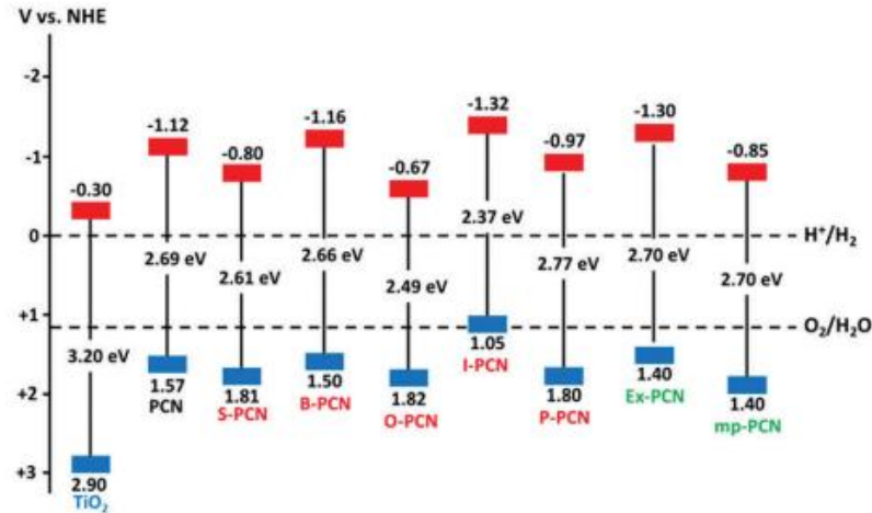
FIGURA 1. 5 – Diagrama de bandas de alguns semicondutores com nitretos de carbono dopados com heteroátomos e os valores de bandgaps . Linhas pontilhadas indicam o potencial para o processo de water splitting .
