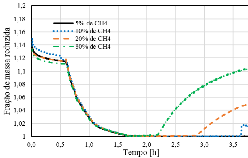
Figura 5.21. Reações a 700 °C com vazão de 50 mL/min, catalisador 2,5%FeMgAl 2 O 4 variando a fração de metano na alimentação.
