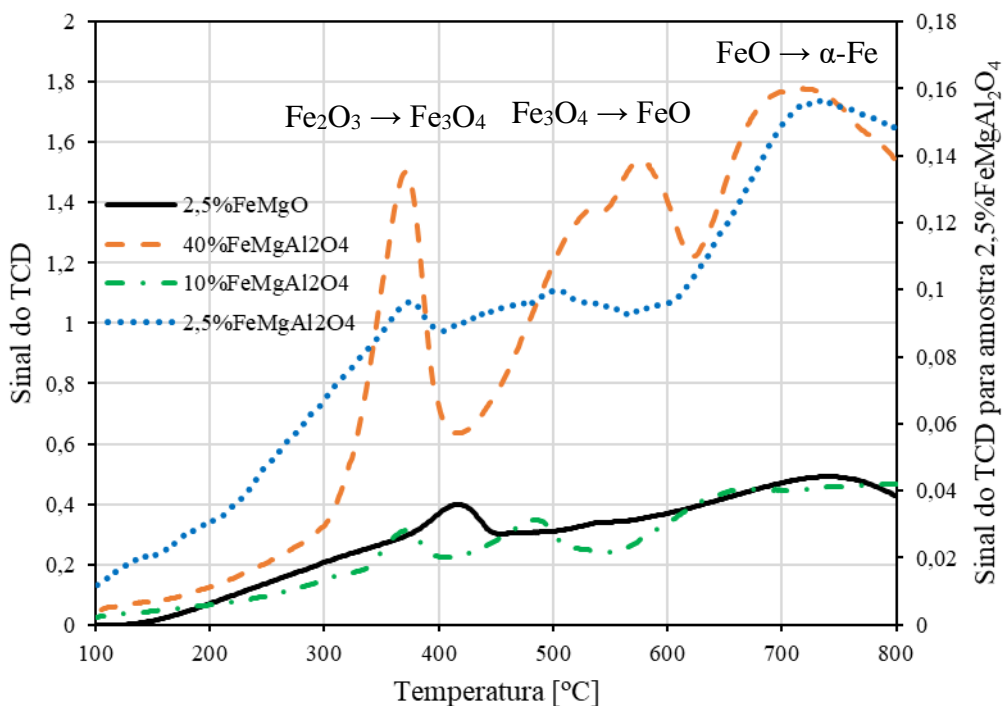
Figura 5.8. TPR dos catalisadores estudados.
