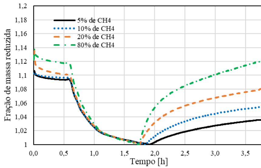
Figura 5.20. Reações a 750 °C com vazão de 50 mL/min, catalisador 2,5%FeMgAl 2 O 4 variando a fração de metano na alimentação.
