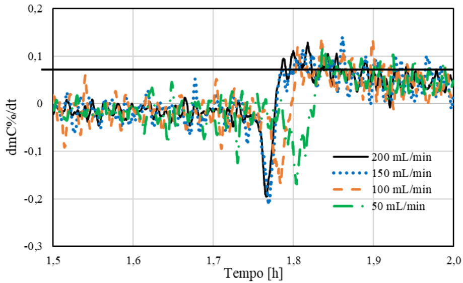
Figura 5.16. Taxas de reação sobre catalisador 2,5%FeMgAl 2 O 4 variando a vazão.
