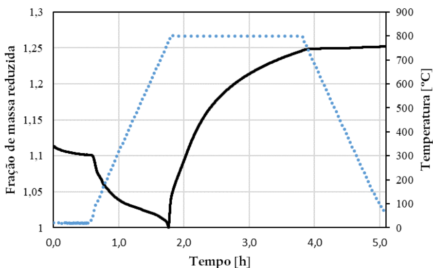
Figura 4.1. Exemplo de resultado obtido na termobalança, fração de massa reduzida (em preto sólido) e temperatura do sistema (azul pontilhado).
