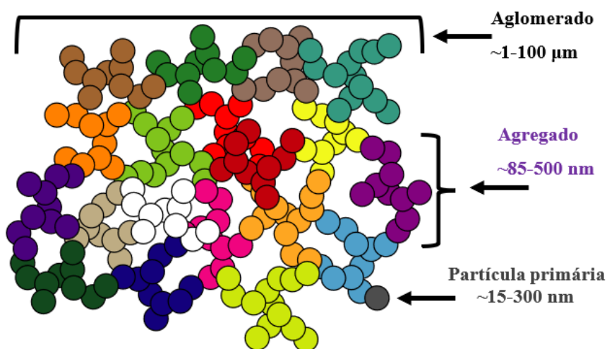
Figura 2.5. Estrutura do negro de fumo com diâmetros típicos dos componentes.
