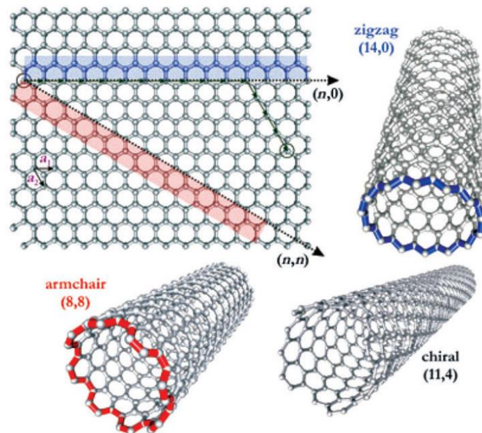
Figura 2.3. Conformações dos nanotubos baseados no vetor quiral.
