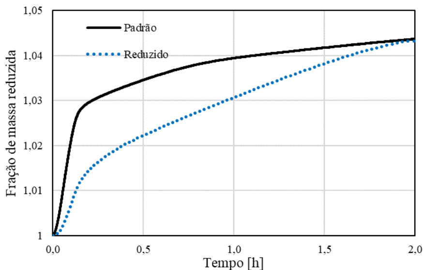
Figura 5.10. Reações com o catalisador 2,5% FeMgO com e sem redução sob H_2 .
