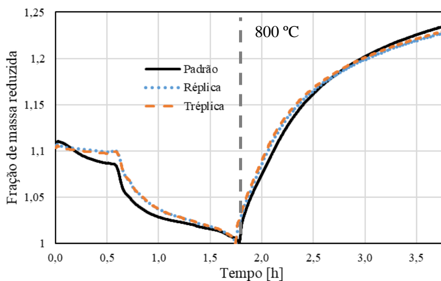
Figura 5.11. Reações com 10 mg do catalisador 10%FeMgAl 2 O 4 a 800 °C, com 10% de metano na alimentação com vazão total de 100 mL/min.
