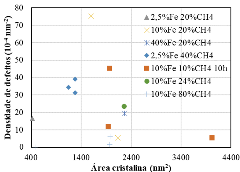
Figura 5.28. Caracterização dos materiais quanto à densidade de defeitos e área cristalina.
