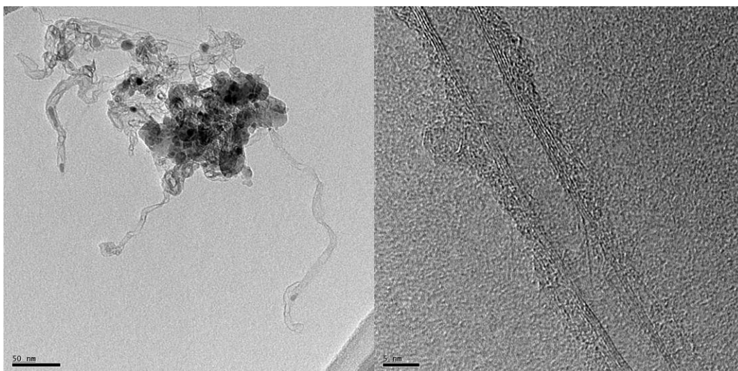
Figura 5.31. Imagens de microscopia do catalisador 2,5%FeMgAl 2 O 4 reagido.
