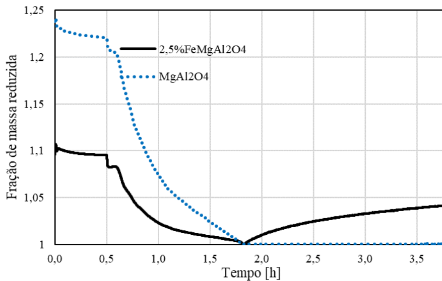
Figura 5.17. Reações sobre o catalisador 2,5%FeMgAl 2 O 4 e suporte MgAl 2 O 4 a 800 °C com vazão de 50 mL/min, e fração de metano 0,05.
