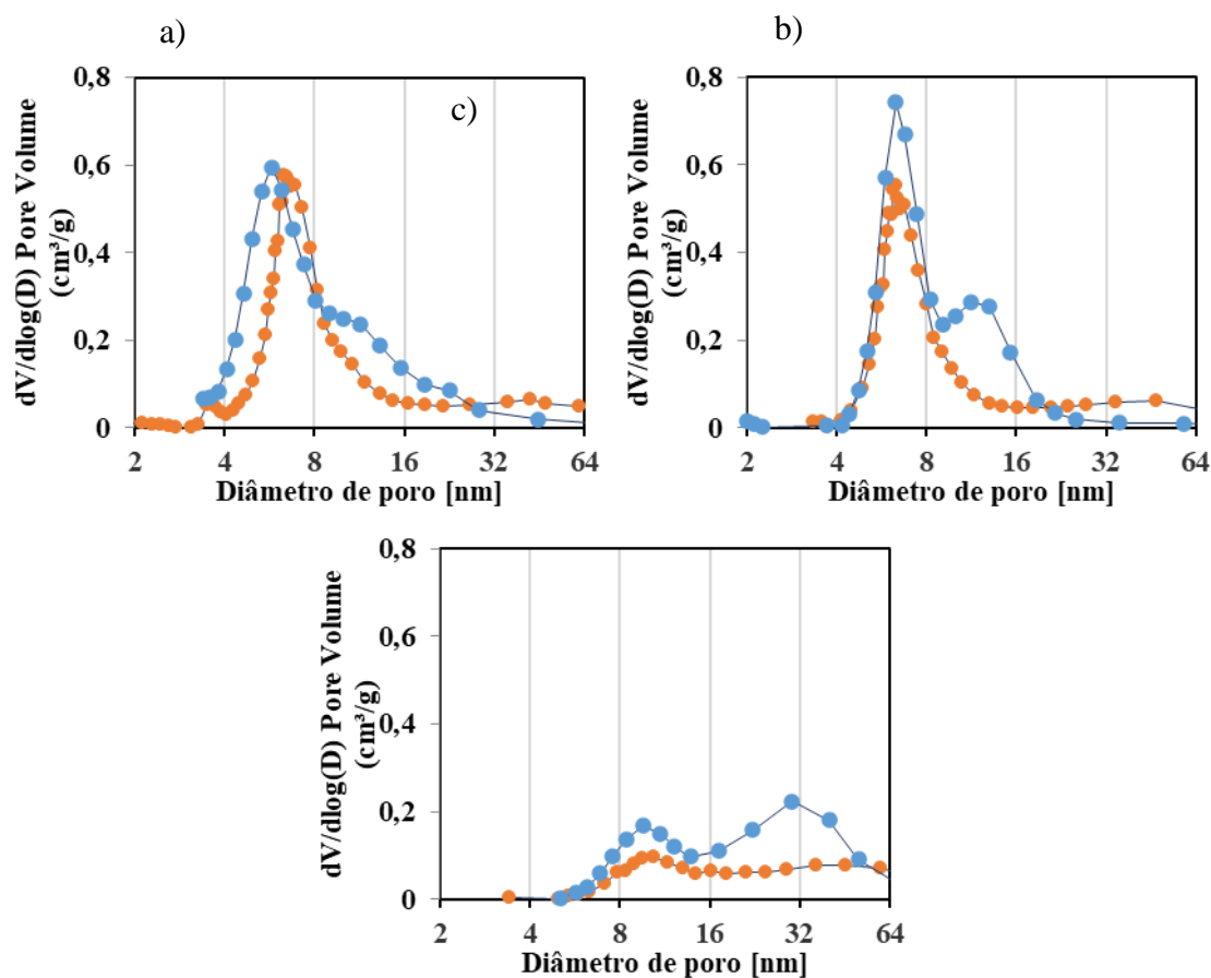
Figura 5.26. Distribuição de diâmetro de poros do catalisador fresco (azul) e usado (laranja) do (a) catalisador 2,5%FeMgAl 2 O 4 , (b) 10%FeMgAl 2 O 4 e (c) 40%FeMgAl 2 O 4 .
