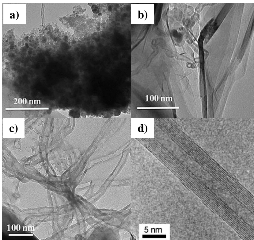
Figura 2.6. Imagens de MET de carbono nanométrico, a) esferas, b) grafite e corrente, c) nanotubos de carbono e d) nanotubo em alta definição.
