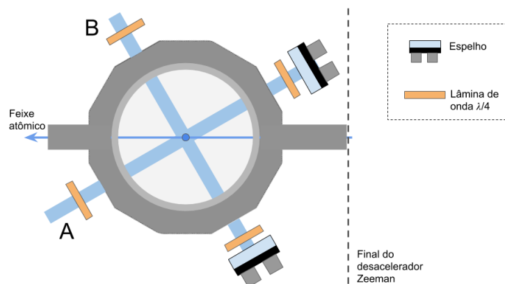
Figura 17: Esquema da câmara de ciência mostrando a entrada dos feixes utilizados para a produção das duas MOTs. Os feixes em azul representam o caminho percorrido pelos feixe do MOT, entram por A/B e sendo refletidos no espelho.
