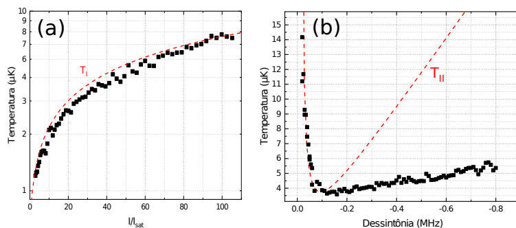
Figura 24: Evolução da temperatura: (a) Como função da saturação à esquerda para dessintonia de \Delta - 500 kHz. (b) Como função da dessintonia para parâmetro de saturação s = 430 . O regime II é satisfeito apenas para \Delta < 0.16 MHz, assim não é esperado uma concordância experimental para \Delta > 0.16 MHz. Os quadrados representam medidas experimentais e as curvas em vermelho tracejadas os valores esperado dados por (5.15) e (5.16), para as figura (a) e (b), respectivamente.
