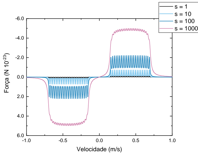
Figura 21: Força resultante do caso unidimensional para espectro multi-cromático. Cálculo feito com uma componente de frequência a cada 35 kHz com dessintonia indo de - 1 MHz até - 200 kHz. O parâmetro de saturação s corresponde a saturação do total do feixe, isto é, cada componente tem saturação s_c \approx 1/28
