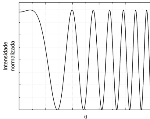
Figura 5: Intensidade resultante do espalhamento de luz por um átomo em frente ao espelho.
