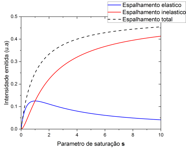
Figura 1: Comparação entre quantidade de luz espalhada de maneira elástica e inelástica como função da intensidade de saturação
