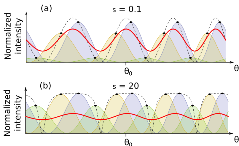
Figura 7: Diminuição do contraste das franjas de interferência com o aumento da intensidade. Na figura as curvas preenchidas representam o espalhamento de átomos em diferentes posições da onda estacionária, e a curva vermelha as franjas resultantes. Figura extraída de (21).
