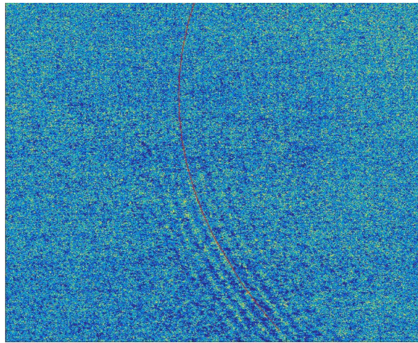
Figura 37: Imagens das franjas de interferência. A curva vermelha representa o círculo sobre o qual todos os pontos são integrados para produzir a curva como função do ângulo.
