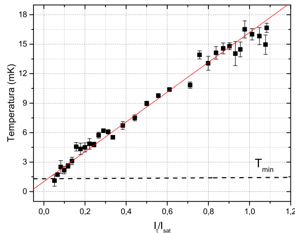
Figura 20: Evolução da temperatura do MOT-Azul para diferentes potências totais no MOT-Azul. Os quadrados são medidas de temperatura, e a curva em vermelho representa um ajuste de uma função linear
