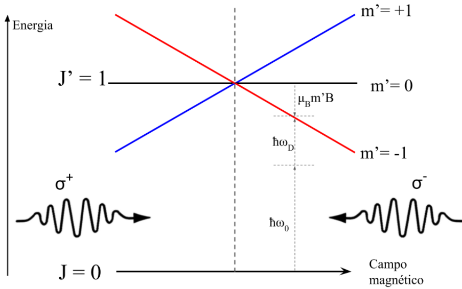
Figura 19: Configuração do MOT mostrando os desvios causados pelo campo magnético e os feixes com suas respectivas polarizações favorecendo transições diferentes para B > 0 e para B < 0 . A dessintonia do feixe laser em relação a transição atômica é compensada pelo desvio Doppler com frequência \omega_D e pelo Efeito Zeeman.
