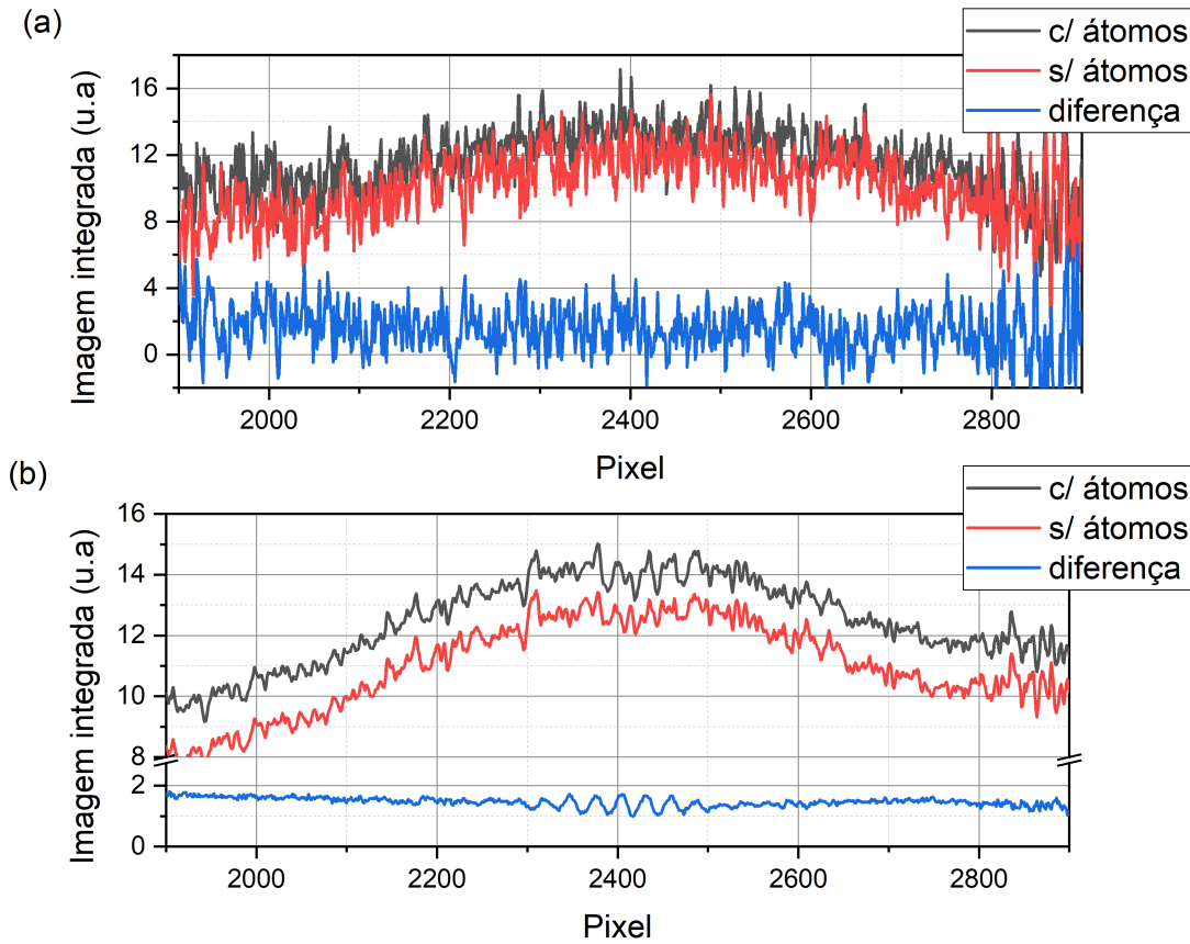
Figura 38: Redução da flutuação na intensidade espalhada devido à média sobre várias realizações para uma mesma configuração de potência. (a) Curvas integradas sobre apenas 1 realização; (b) Curvas integradas sobre 1000 realizações.
