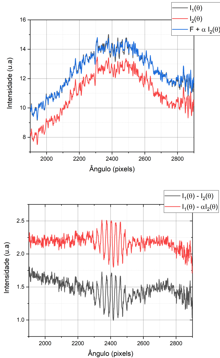
Figura 39: Comparação do ajuste linear nas franjas de interferência. (a) Comparação das imagens 1 e 2 integradas no radialmente. Como podemos ver a curva ajustada azul concorda muito bem com a I_1(\theta) na região fora das franjas de interferência. (b) As franjas após o ajuste linear aparecem sobre um fundo de intensidade mais constante. Medidas realizadas para \theta_0 = 3.13^\circ , e potência de 1 mW.
