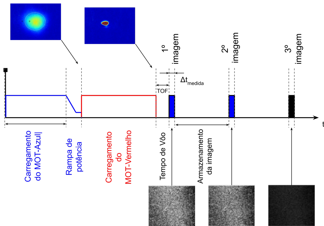
Figura 35: Sequência experimental para realização da medida de espalhamento. Os inserts superiores são imagens de absorção da nuvem em diferentes etapas do processo de resfriamento. As cores representam cores falsas apenas para melhor visualização.
