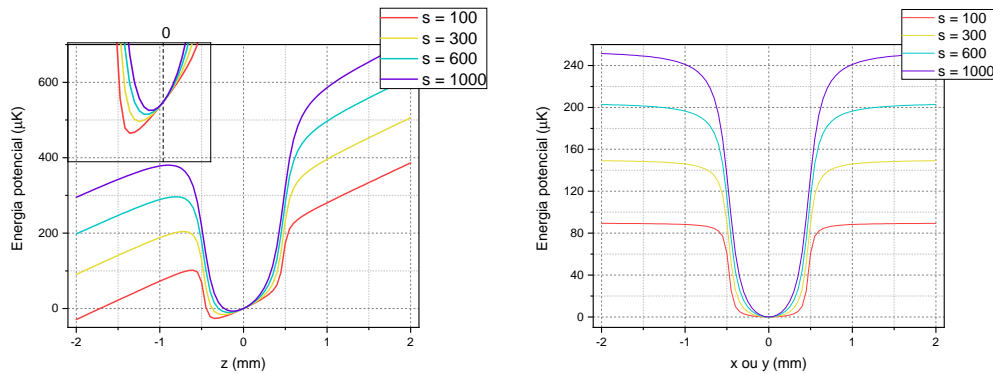
Figura 25: Potencial para o regime II: (a) Podemos ver que com o aumento da potência, a posição de equilíbrio volta em direção a origem e o potencial vai se tornando cada vez mais harmônico com o aumento do parâmetro de saturação; (b) O mesmo ocorre para o potencial no plano x - y , que vai se tornando harmônico e cada vez mais confinante.
