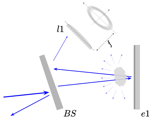
Figura 26: Montagem experimental do interferômetro com elementos óticos. Os feixes de laser são as setas azuis contínuas, enquanto a luz espalhada pelos átomos está representada pelas setas tracejadas em azul. As legendas para a imagem são: BS = divisor de feixe; e1 = espelho; l1 = lente com distância focal f para conjugação das franjas.
