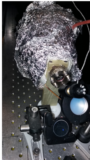
Figura 11: Célula de espectroscopia utilizada como referência de frequência para sistema laser azul. Essa célula é aquecida por uma resistência que dissipa \approx 36 W e esta coberta por algodão e lã de vidro para isolamento térmico. Além do Estrôncio metálico, a célula também é preenchida com 1 mbar de argônio, que age como um buffer gas para evitar a deposição do metal nas janelas (25)
