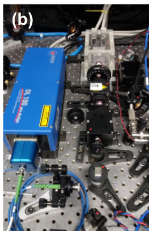
Figura 15: (a) Esquema do sistema vermelho de laser; (b) A caixa azul é o laser vermelho de diodo com uma saída acoplada diretamente a uma fibra. A caixa transparente de acrílico é o laser de diodo utilizado para o Injection Lock ; (c) A cavidade preta é a cavidade ultra-estável que serve como referência para o laser vermelho
