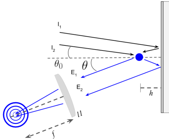
Figura 3: A luz espalhada por um átomo a uma distância h do espelho é coletada pela lente l1 de foco f , e interfere no plano focal dessa lente gerando franjas de interferência.
