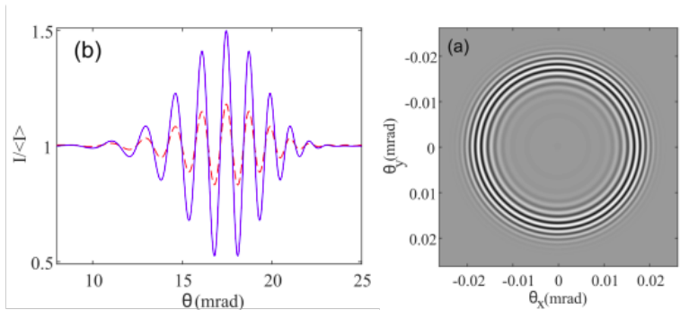
Figura 6: Franjas de interferência resultantes do espalhamento de radiação por uma nuvem atômica na frente de um espelho. Figura extraída de (24).
