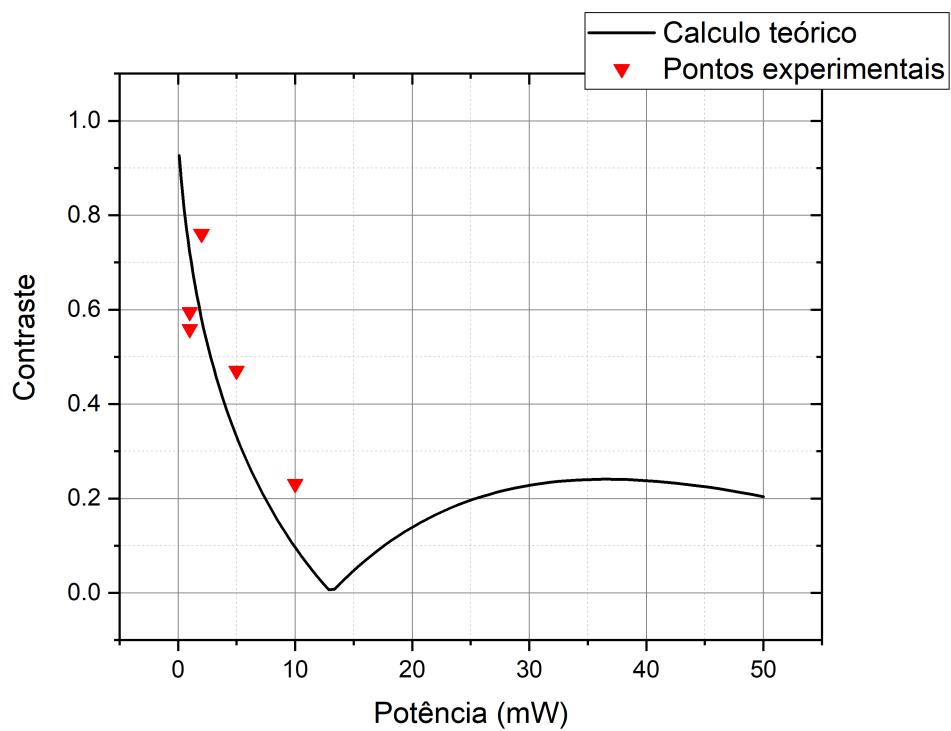
Figura 40: Comparação entre previsão teórica e pontos experimentais obtidos para curva do contraste como função da potência. Os pontos obtido são para potências de 1 mW; 2 mW; 5 mW e 10 mW. No momento estamos estimando os valores para as barras de erro.
