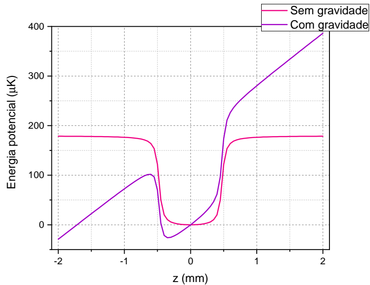
Figura 22: Efeito da gravidade no potencial criado pela força ótica em z no regime I. O potencial que tem uma forma do tipo caixa se deforma no eixo z alterando a posição de equilíbrio dos átomos. Potencial calculado a partir da integral de caminho da força (5.14).
