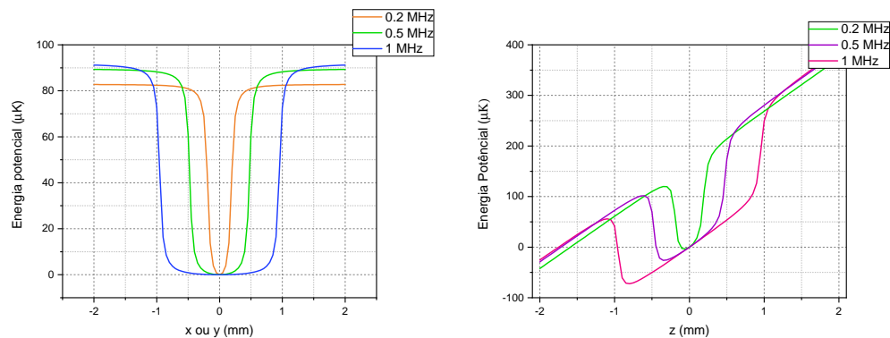
Figura 23: Potencial no regime I. (a) Potencial no plano x - y para diferentes dessintonias: Como podemos ver nesse caso temos um potencial do tipo caixa, cuja largura depende da frequência utilizada. (b) Potencial no eixo z para diferentes dessintonias: A posição de equilíbrio do depende da frequência utilizada.
