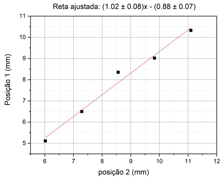
Figura 30: Calibração da posição do espelho virtual utilizando a separação entre franjas. Posição 1 é a estimativa da posição do espelho segundo a separação das franjas, enquanto posição 2 é a posição medida externamente a partir de uma origem estimada com base na posição das lentes e espelho.
