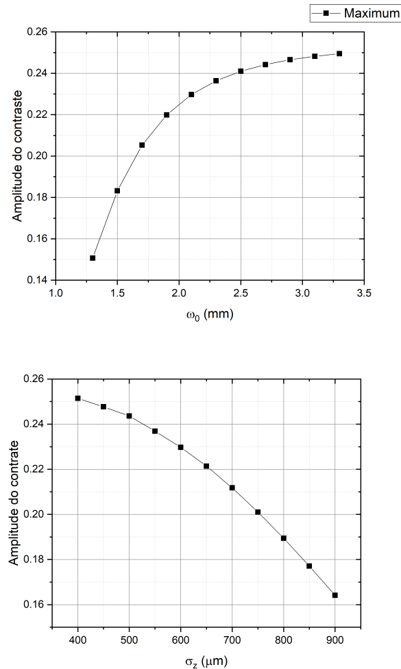
Figura 32: Simulações da amplitude da oscilação do contraste. (a) Para uma nuvem com \sigma_z = 600 \mu\text{m} e diferentes tamanhos do feixe. (b) Para um feixe com \omega_0 = 2.1 mm, e diferentes tamanhos da nuvem.
