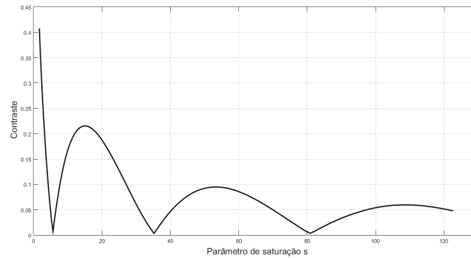
Figura 8: Contraste resultante para o espalhamento em alta intensidade
