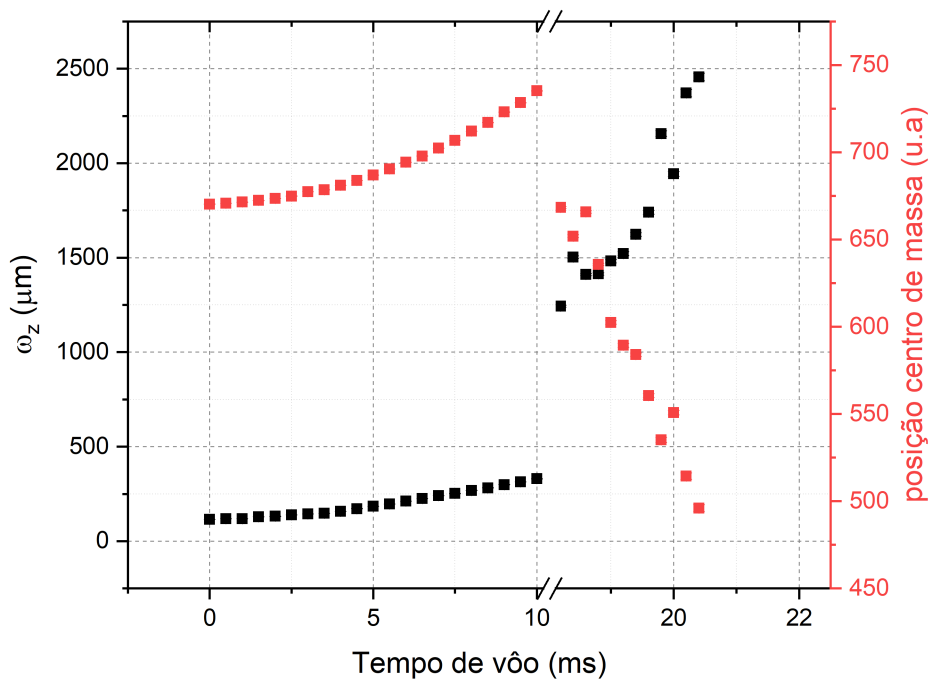
Figura 36: Evolução da nuvem no eixo z após um pulso \delta t = 2 \mu s e potência de 10 mW. O espaço vazio de pontos no gráfico representa uma região não acessível a observação utilizando imagens de absorção por limitações experimentais.
