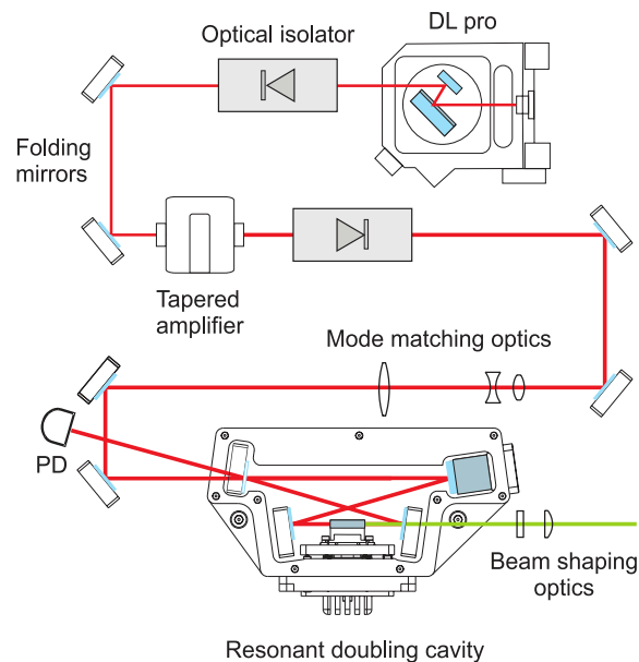
Figura 10: Esquema do laser azul TA-SHG-Pro extraído de (28). O laser verde é igual exceto pela ausência do TA e do isolador óptico logo após a saída do amplificador. A necessidade de uma menor potência de re-bombeio justifica a ausência do amplificador.
