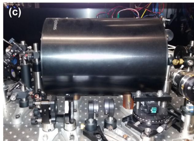
Figura 15: (a) Esquema do sistema vermelho de laser; (b) A caixa azul é o laser vermelho de diodo com uma saída acoplada diretamente a uma fibra. A caixa transparente de acrílico é o laser de diodo utilizado para o Injection Lock ; (c) A cavidade preta é a cavidade ultra-estável que serve como referência para o laser vermelho
