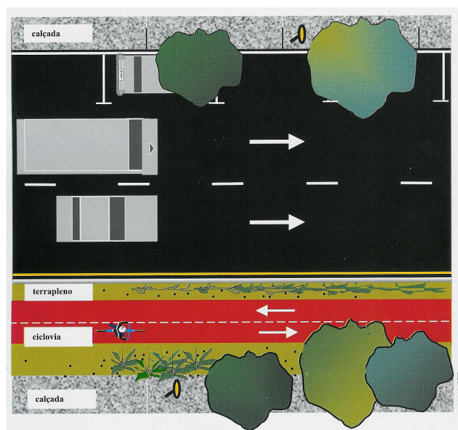
Figura 2.2: Esquema de uma ciclovia paralela ao sistema viário – Fonte: Geipot, 2001a
